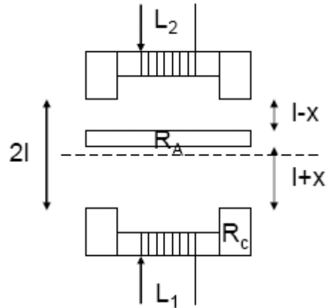
Hình 2.41: Cấu trúc cảm biến vi sai
