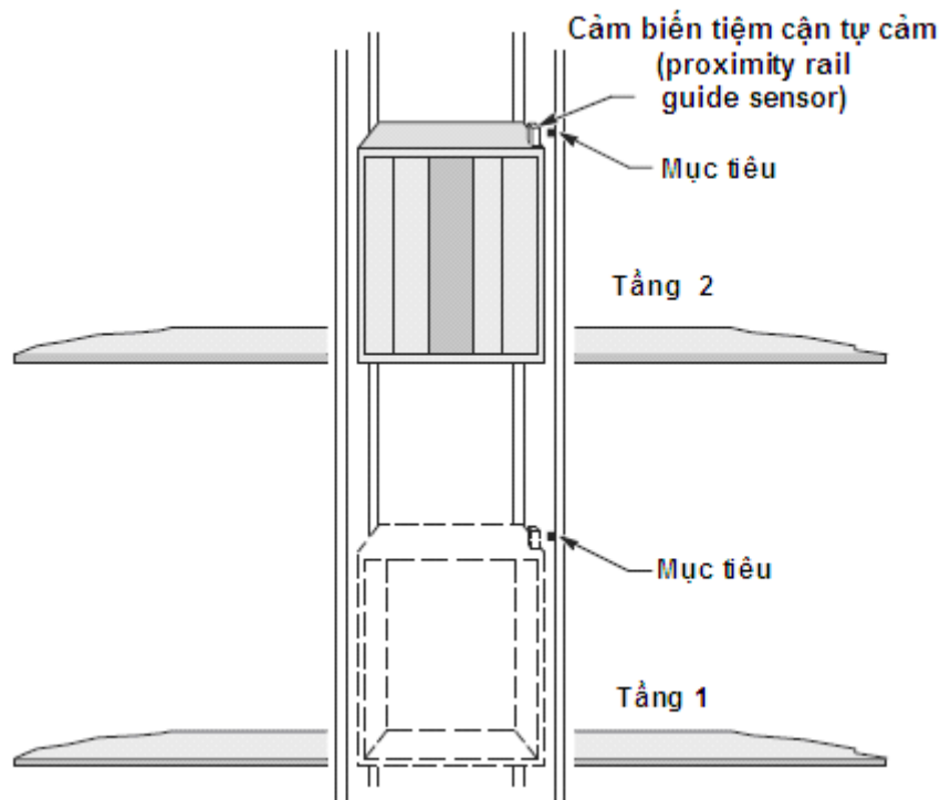
Xác định vị trí của thang máy
