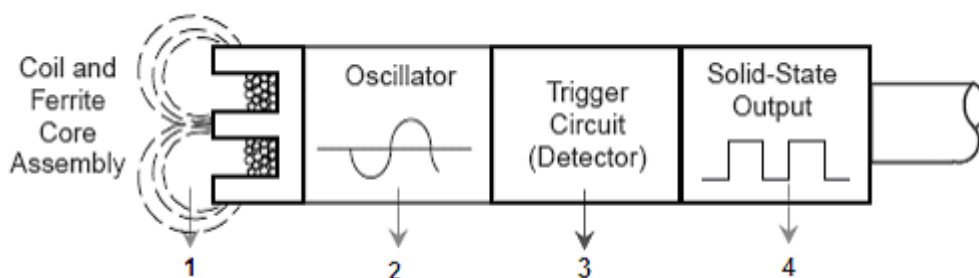
Hình 2.6: Cấu trúc của cảm biến
