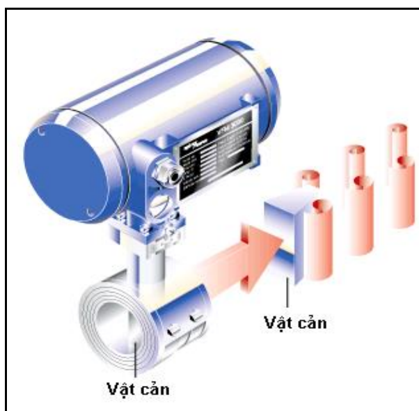
Hình 3.22: Cảm biến đo lưu lượng với nguyên tắc tần số dòng xoáy
