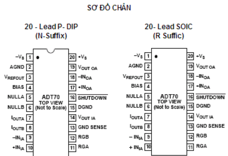
Hình 1.40: Sơ đồ chân ADT 70
