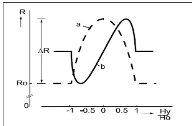
Hình 4.17: Ảnh hưởng của barber poles
