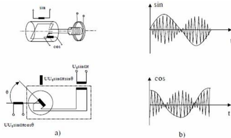
Hình 4.20 Sơ đồ nguyên lý máy đo góc tuyệt đối
