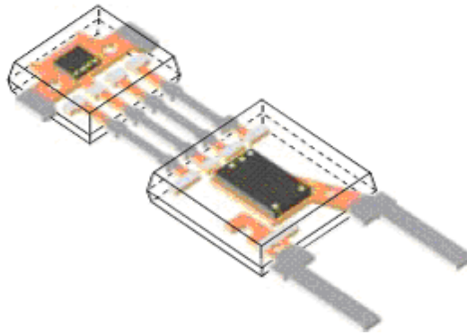
Hình 4.22: Cấu trúc loại cảm biến KMI
