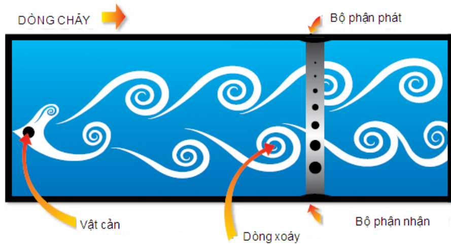
Hình 3.27: Kỹ thuật đo dùng Sóng siêu âm
