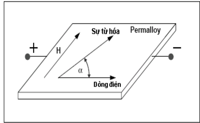
Hình 4.15: Hiệu ứng điện trở từ trên permalloy
